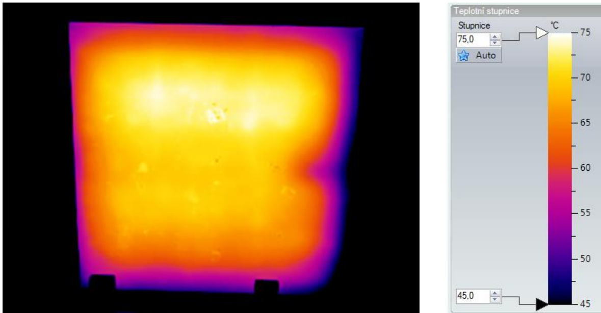
Obr.č.13 – termovízny snímok priebehu teplôt na povrchu panela po 60 minútach prevádzky a teplote okolia 20 °C. Vpravo je zobrazená teplotná stupnica v rozsahu 45 až 75°C.
