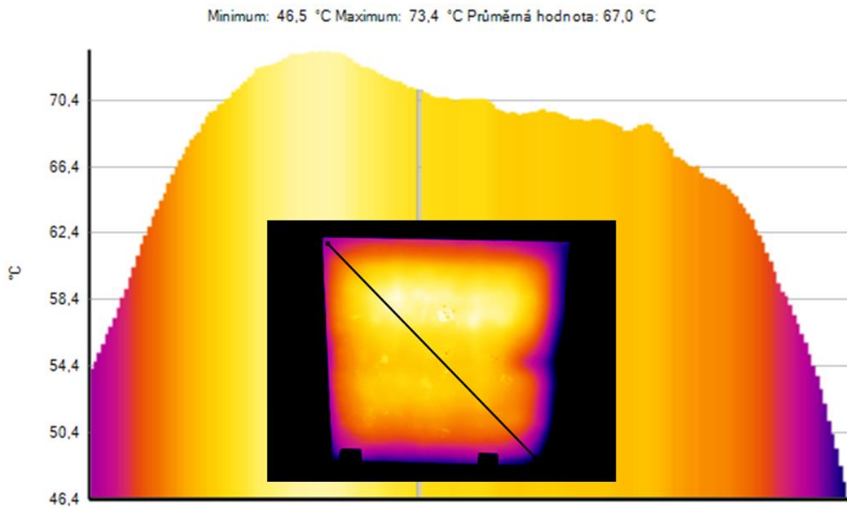
Obr.č.14 – termovízny snímok priebehu teplôt na povrchu panela po 60 minútach prevádzky a teplote okolia 20 °C. Teplotný profil panela po uhlopriečke zľava zhora smerom doprava dole. Minimálna teplota na okraji panela = 46,5°C, maximálna teplota = 73,4°C, priemerná teplota po zvolenej uhlopriečke = 67,0°C.
