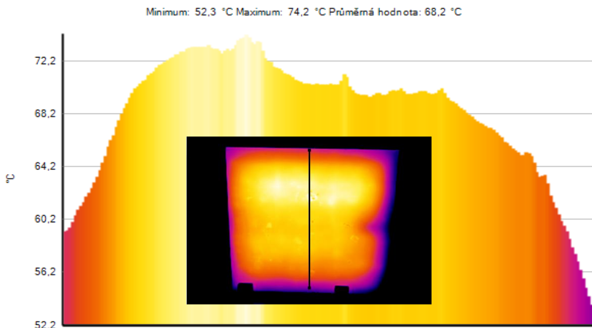
Obr.č.15 – termovízny snímok priebehu teplôt na povrchu panela po 60 minútach prevádzky a teplote okolia 20 °C. Teplotný profil panela po zvislej osi zhora smerom dole. Minimálna teplota na okraji panela = 52,3°C, maximálna teplota = 74,2°C, priemerná teplota po zvolenej osi = 68,2°C.
