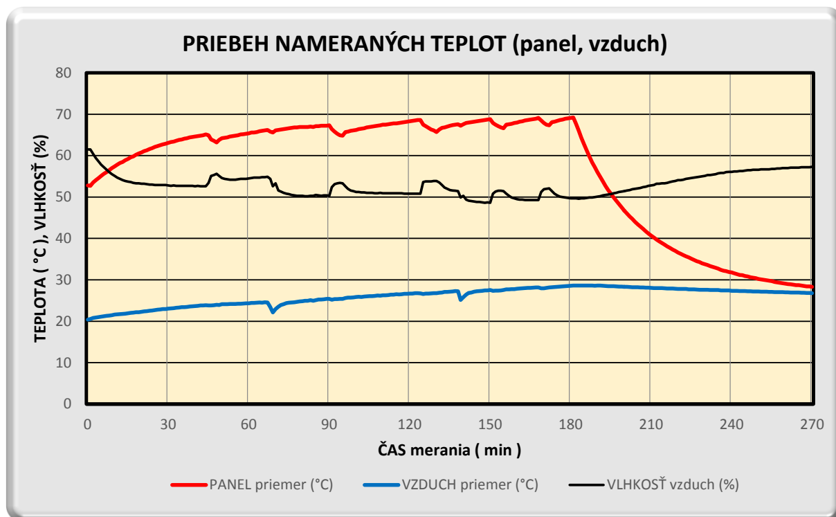
Obr.č.12 – priebeh nameraných hodnôt teploty a relatívnej vlhkosti (teploty sú priemerné)
