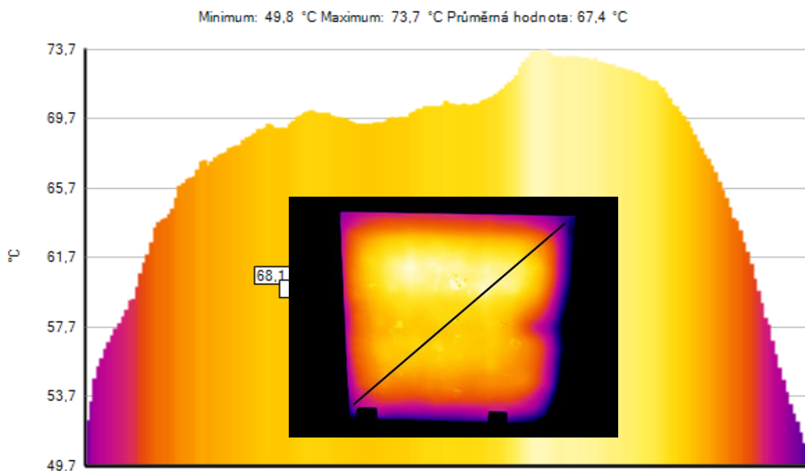
Obr.č.16 – termovízny snímok priebehu teplôt na povrchu panela po 60 minútach prevádzky a teplote okolia 20 °C. Teplotný profil panela po uhlopriečke zľava zdola smerom doprava hore. Minimálna teplota na okraji panela = 49,8°C, maximálna teplota = 73,7°C, priemerná teplota po zvolenej uhlopriečke = 67,4°C.
