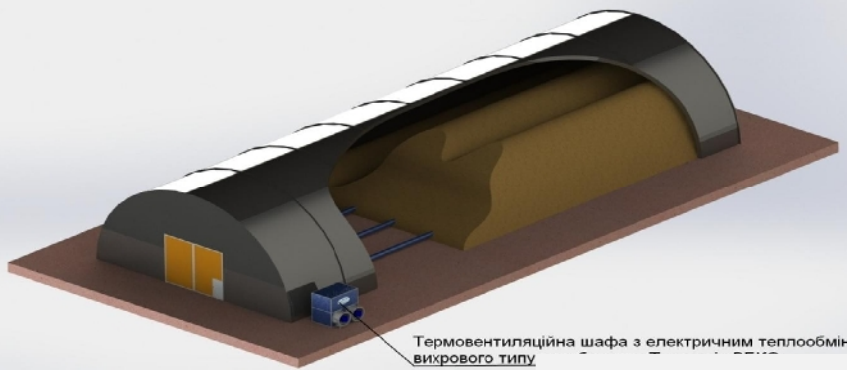
Електричні теплообмінники вихрового типу
